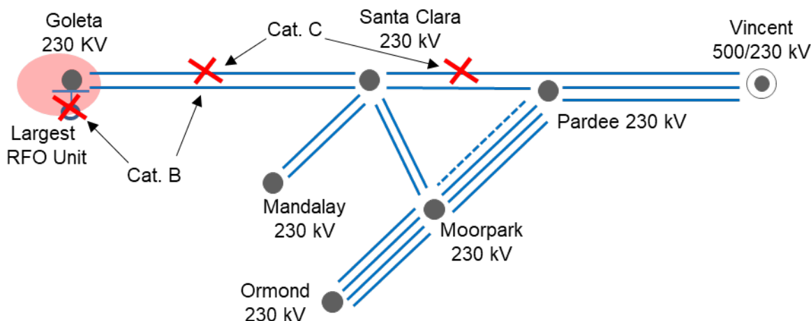
Figure 3.5-79 Goleta LCR Sub-area
