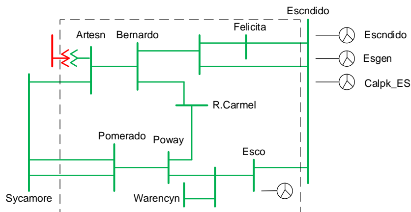
Figure 3.5-92 Esco LCR Sub-area
