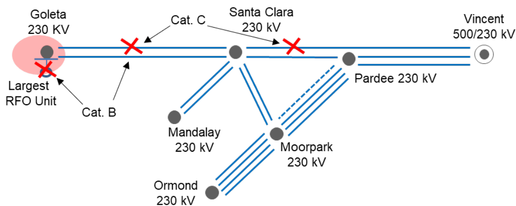
Figure 3.5-79 Goleta LCR Sub-area
