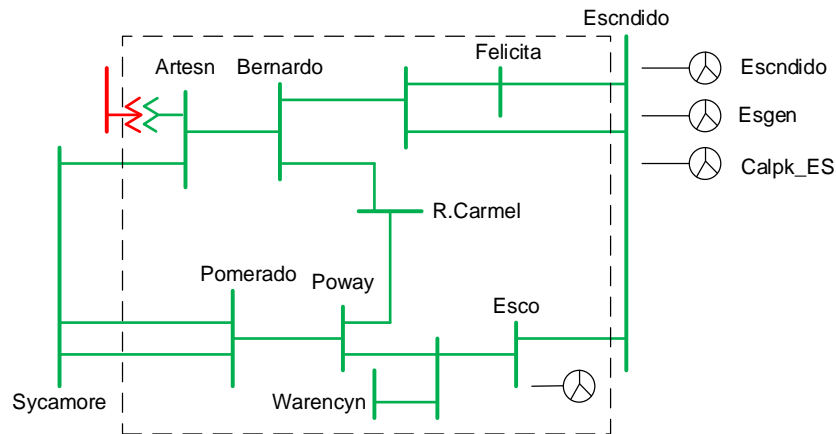
Figure 3.5-92 Esco LCR Sub-area
