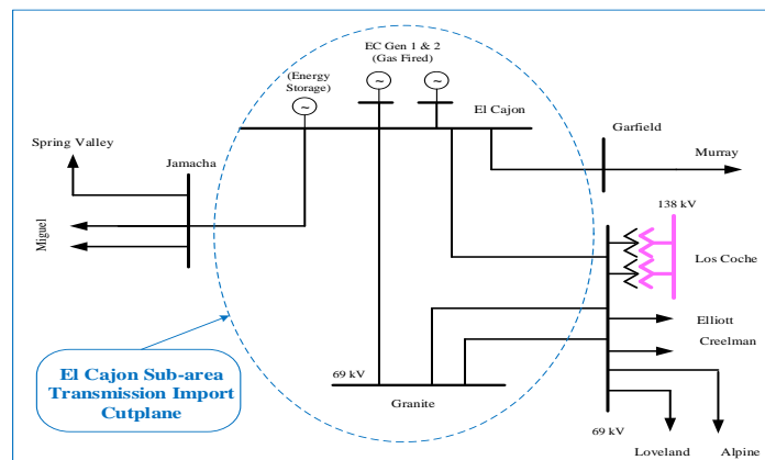
Figure 3.3-107 El Cajon LCR Sub-area
